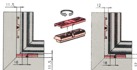
Soporte y enganche de hoja. Cambiando la posición del soporte se varía el desplazamiento horizontal de la hoja en medio milímetro (más o menos).
