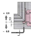
Regulación de hoja en altura. Para regular la hoja aflojar los tornillos del pernio y regular con la llave según se muestra en el detalle. Una vez regulado volver a apretar los tornillos del pernio.
