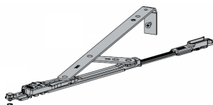
Ref.- 0194-R1 Compás Corto (402 - 750 mm)
