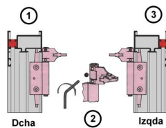
Montaje pernio superior Dcha. e Izqda. Una vez introducido el bulón, poner el tornillo de fijación como muestra la figura 2.
